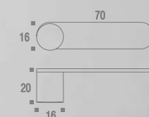
Puxador Rádio P c/ Base Código ZP5444
