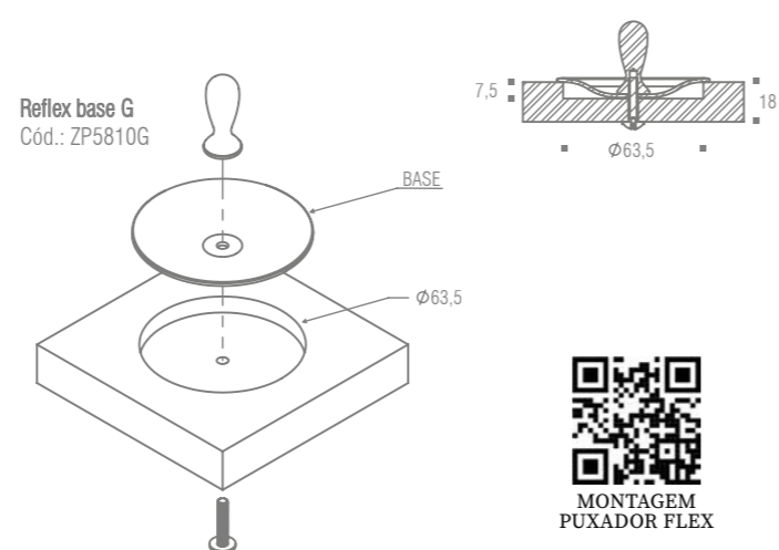
Base Reflex G + Puxador Bali Granado Cód.: ZP5810G | ZP5366
