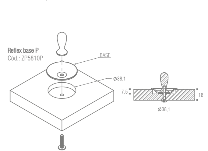
Base Reflex P + Puxador Bali Granado Cód.: ZP5810P | ZP5366
