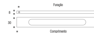
Puxador Magnum Código Furação Comprimento ZP1865 22mm 30mm ZP1934 160mm 174mm ZP1866 224mm 238mm ZP1935 352mm 366mm ZP1936 544mm 558mm
