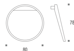
Puxador Afro Código ZP0132 Furação 16mm
