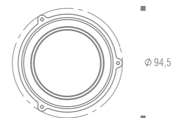
Puxador Dressa Piccolo Pintado Código Diâmetro ZP5803 Ø 94,5mm
