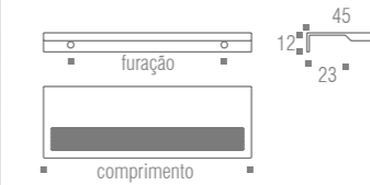
Puxador Citizen Descrição Código Furação Comprimento Citizen P ZP5460 32mm 65mm Citizen G ZP5461 96mm 130mm
